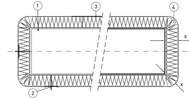
Рисунок 1. Воздуховод с огнезащитным покрытием WIREDMAT в разрезе: 1 – воздуховод, 2 – приварной штифт с шайбой, 3 – покрытие алюминиевой фольгой, 4 – WIREDMAT.
