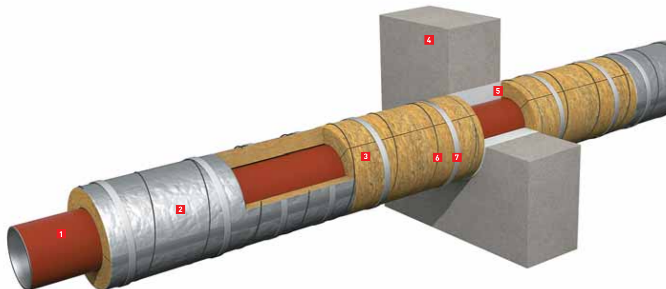
Рисунок 3. Примеры монтажа:
